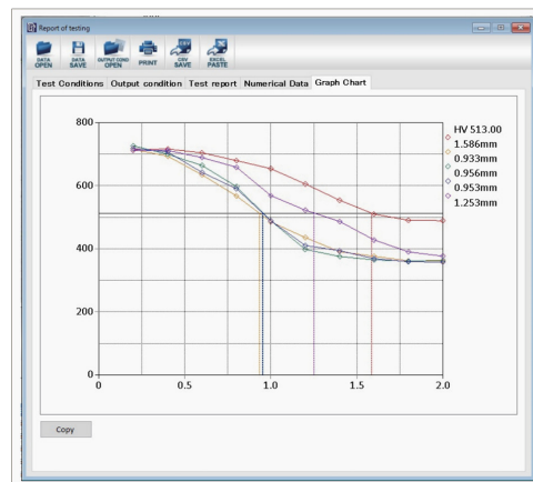
硬化曲線圖
